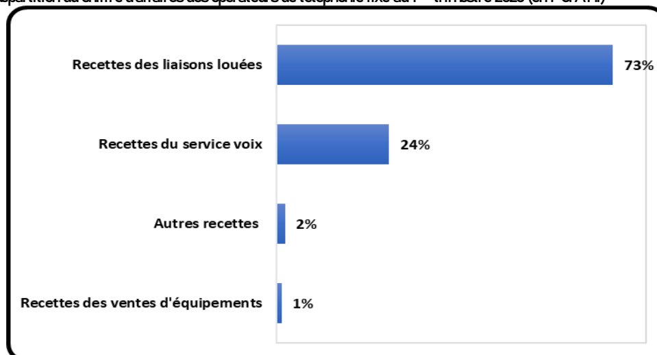
Figure 3: Répartition du chiffre d'affaires par service vendu au 1 er trimestre 2023
